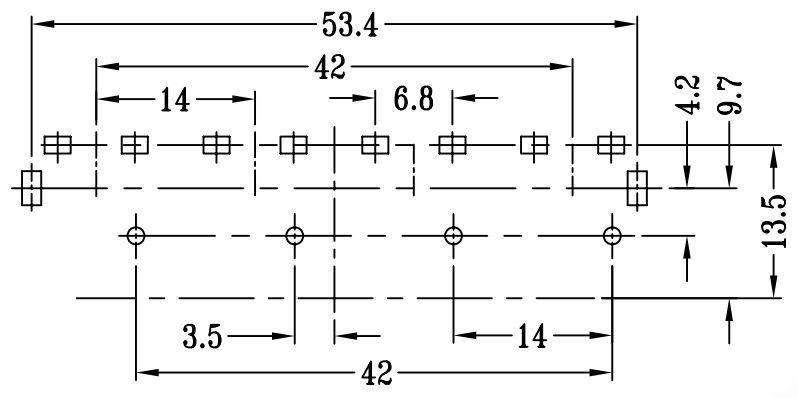
P.C.B LAYOUT
